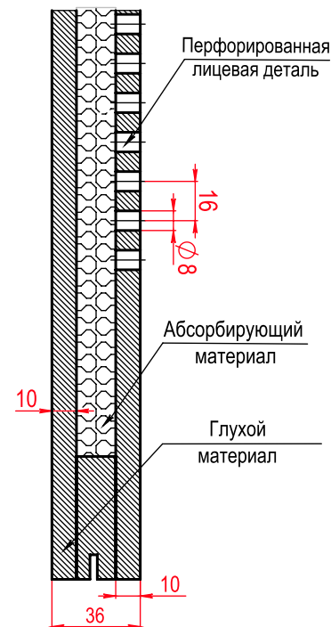
Горизонтальное сечение панели в сборке
